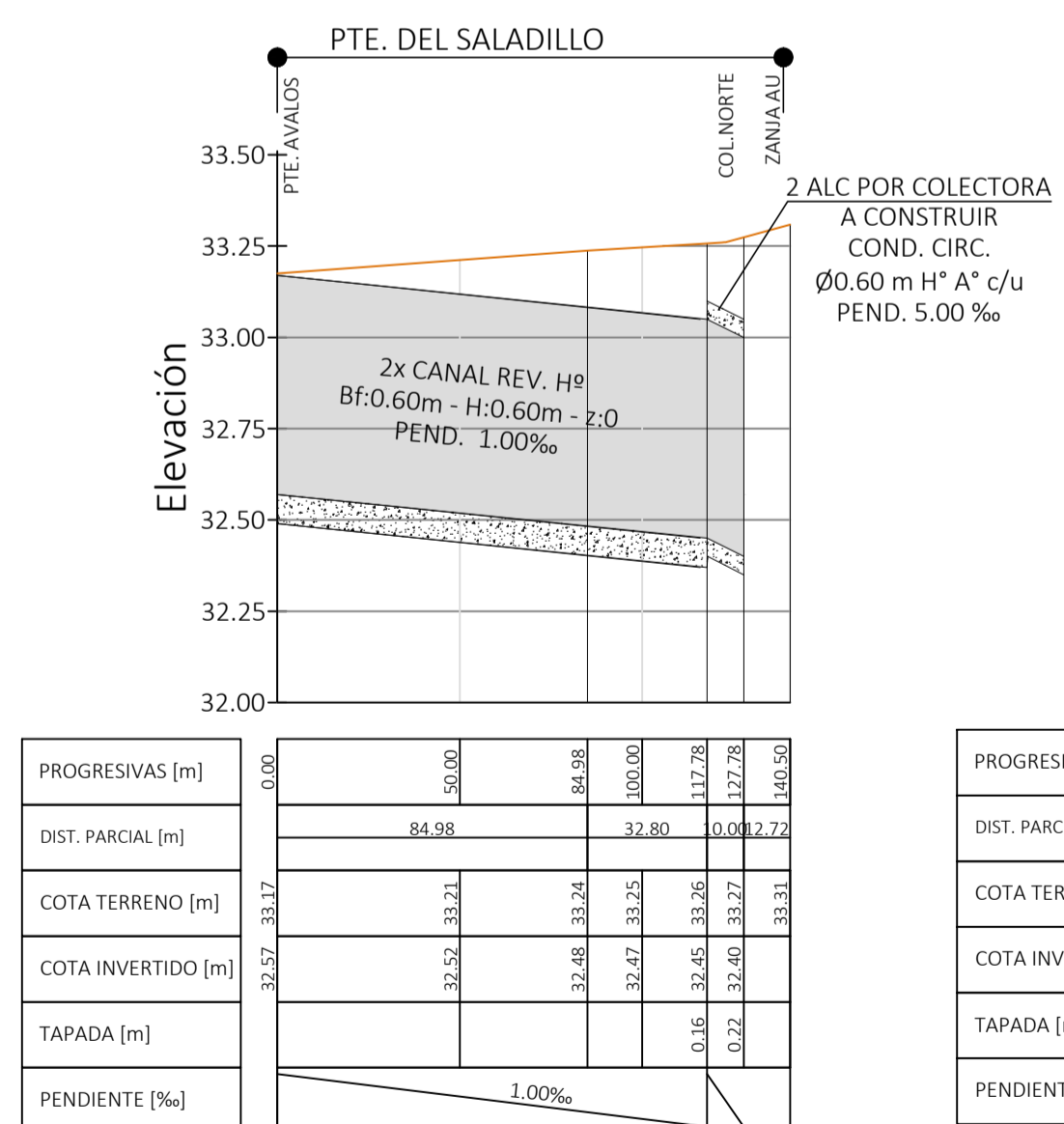
Perfil Longitudinal Ramal 9
