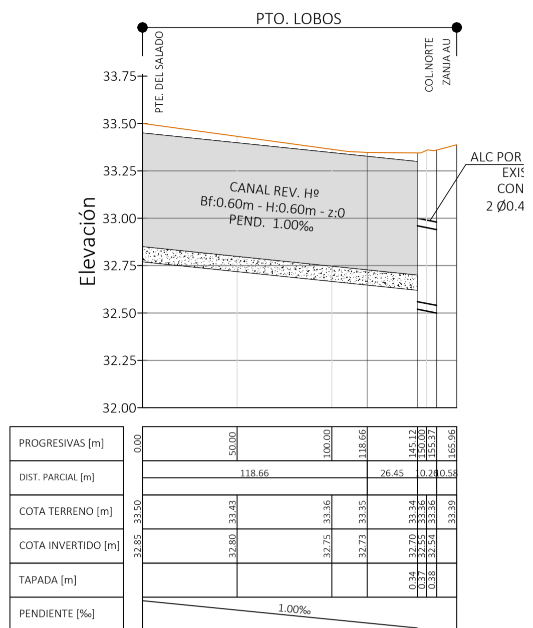
Perfil Longitudinal Ramal 7 izq
