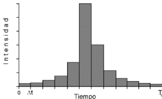
Hietograma de diseño utilizando el Método del Bloque Alterno
