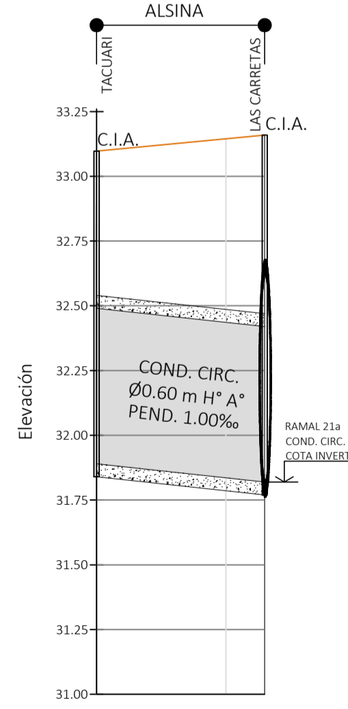
Perfil Longitudinal Ramal 21b
