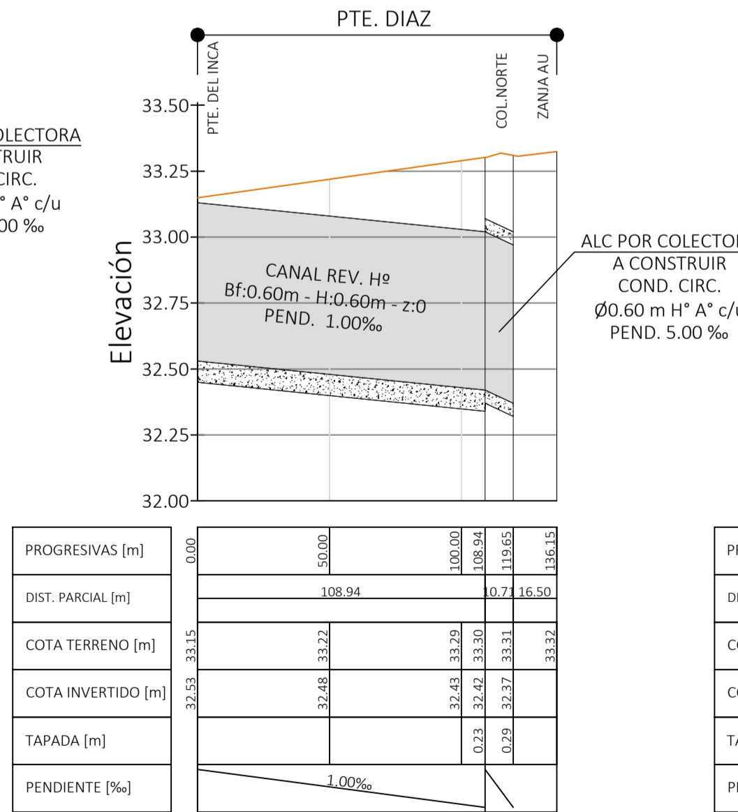
Perfil Longitudinal Ramal 10 der
