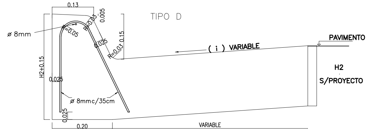
CORDON CUNETA DE ALTURA CONSTANTE
