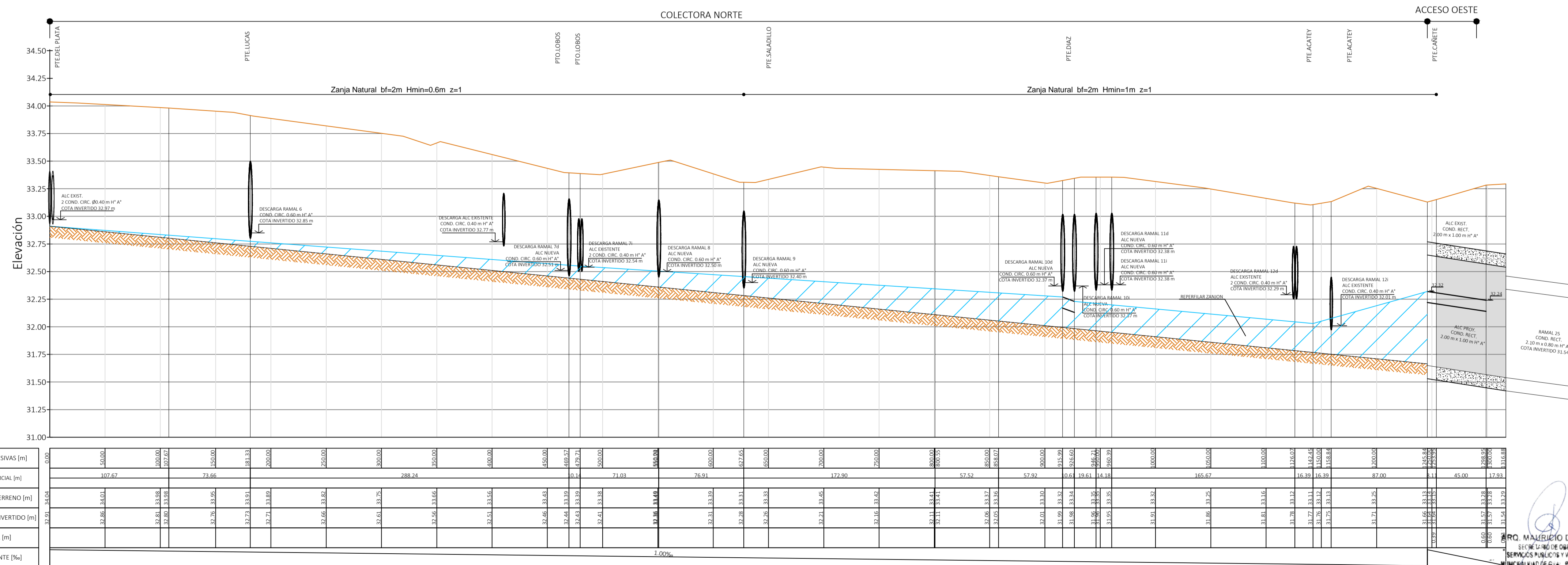
Perfil Longitudinal Ramal 200
