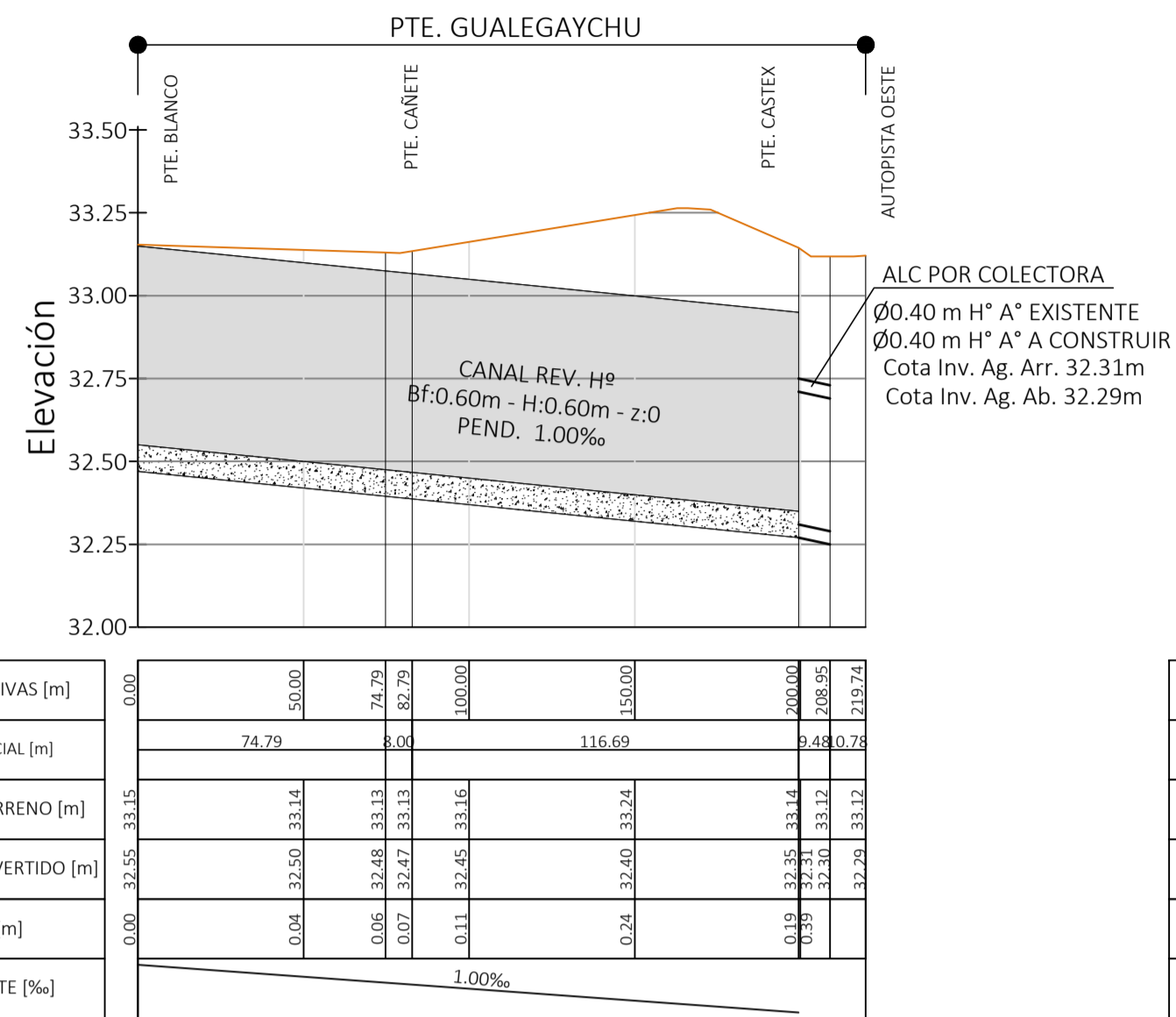
Perfil Longitudinal Ramal 12d
