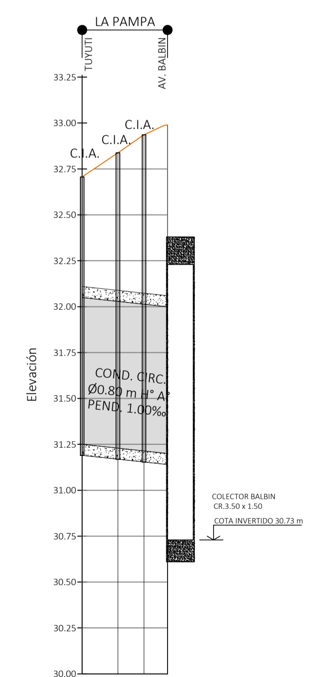
Perfil Longitudinal Ramal 22
