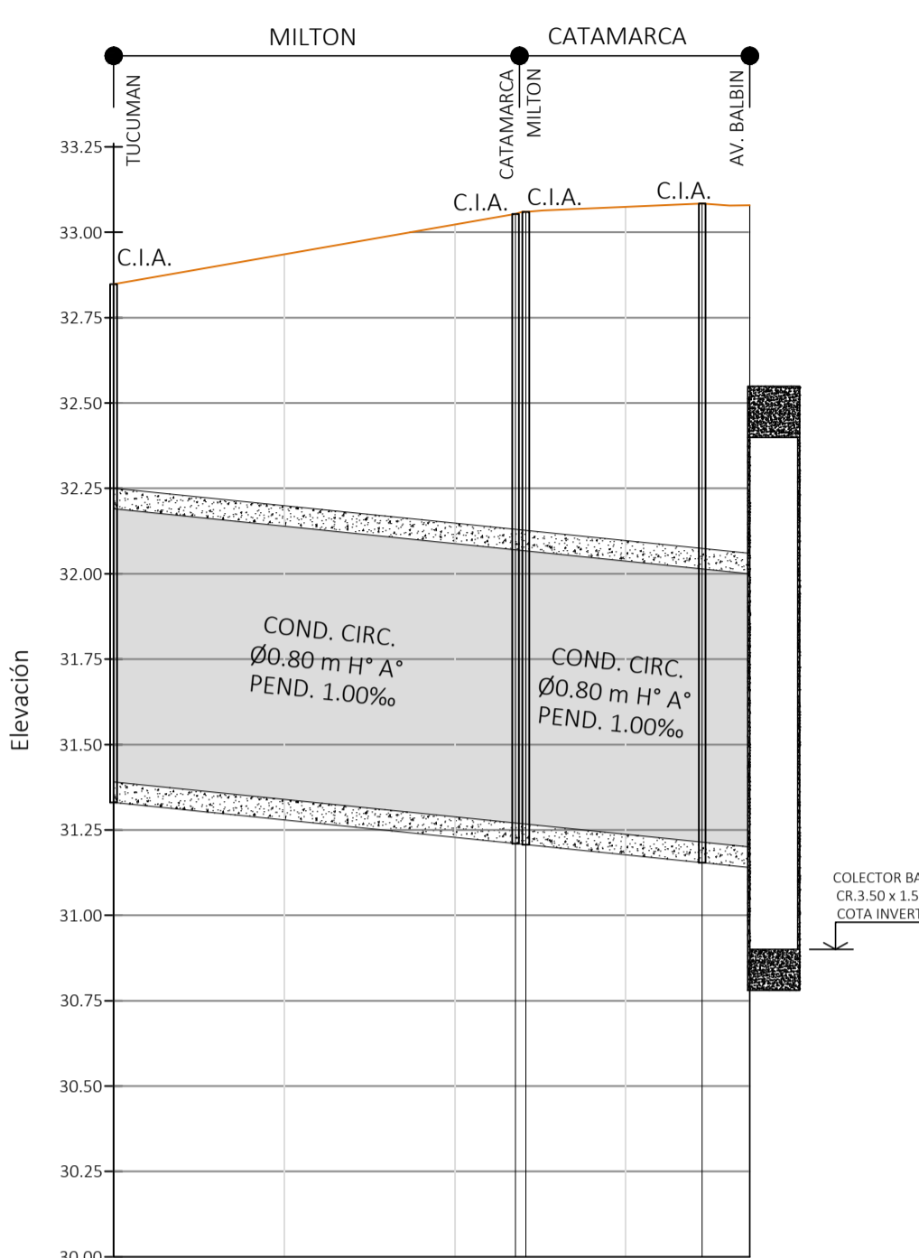
Perfil Longitudinal Ramal 20
