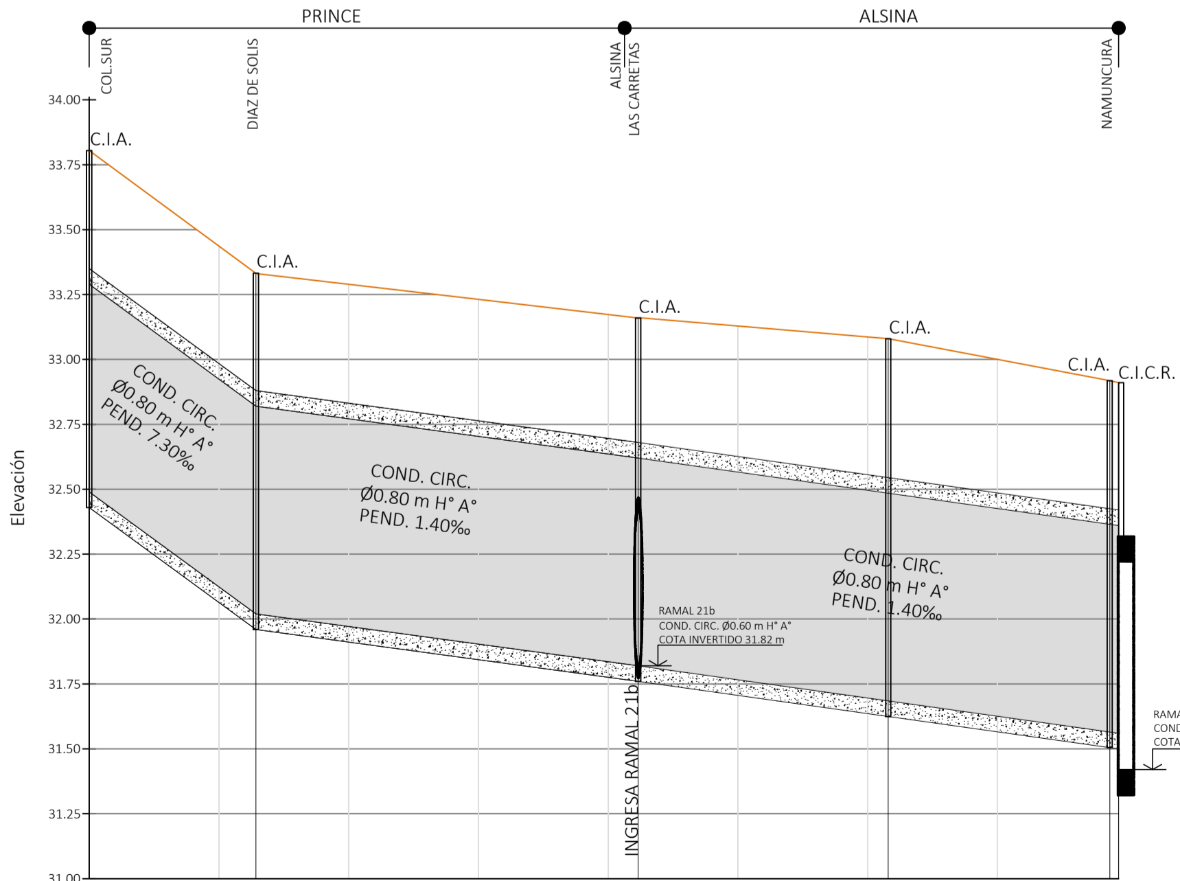
Perfil Longitudinal Ramal 21a
