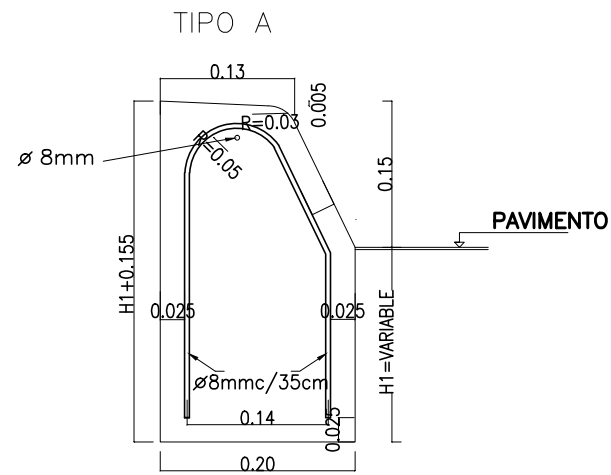
CORDON EMERGENTE DE ALTURA CONSTANTE
