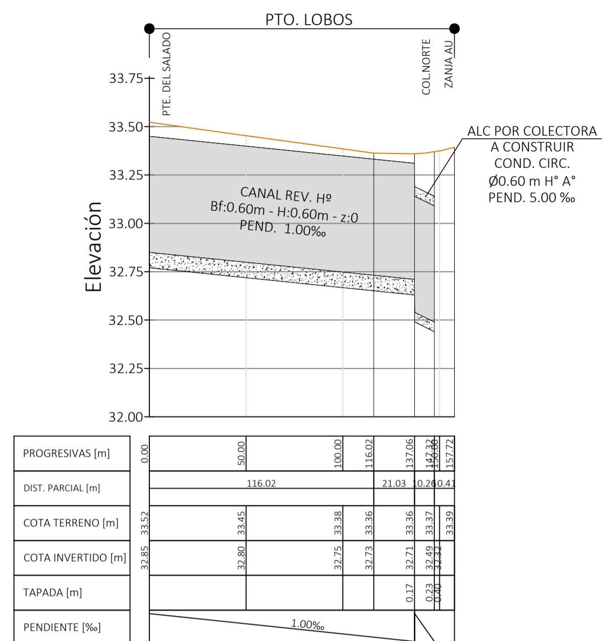
Perfil Longitudinal Ramal 7 der
