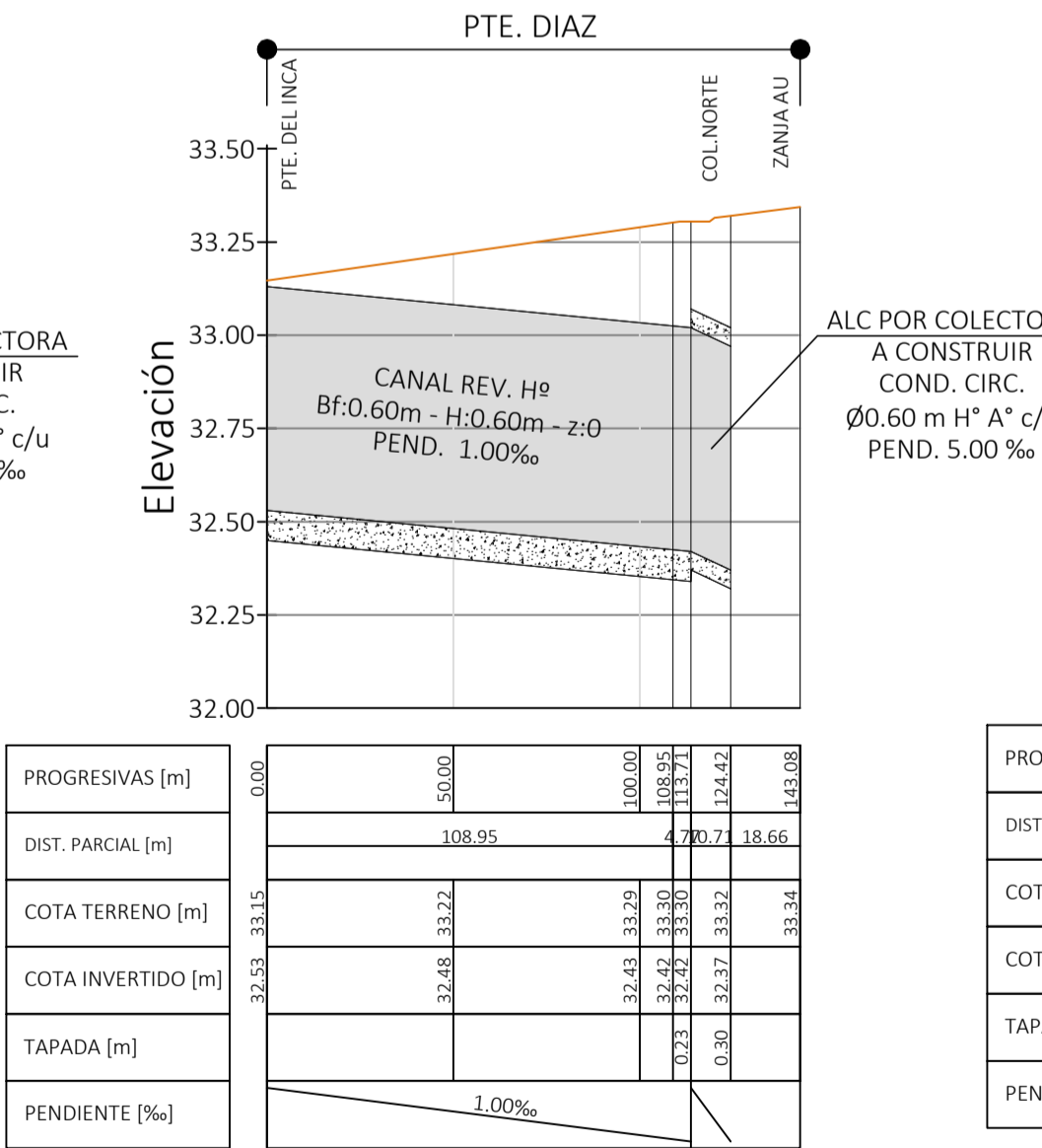
Perfil Longitudinal Ramal 10 izq
