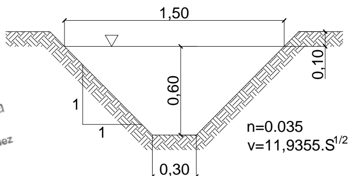
Nivel de servicio de zanja sin revestir
