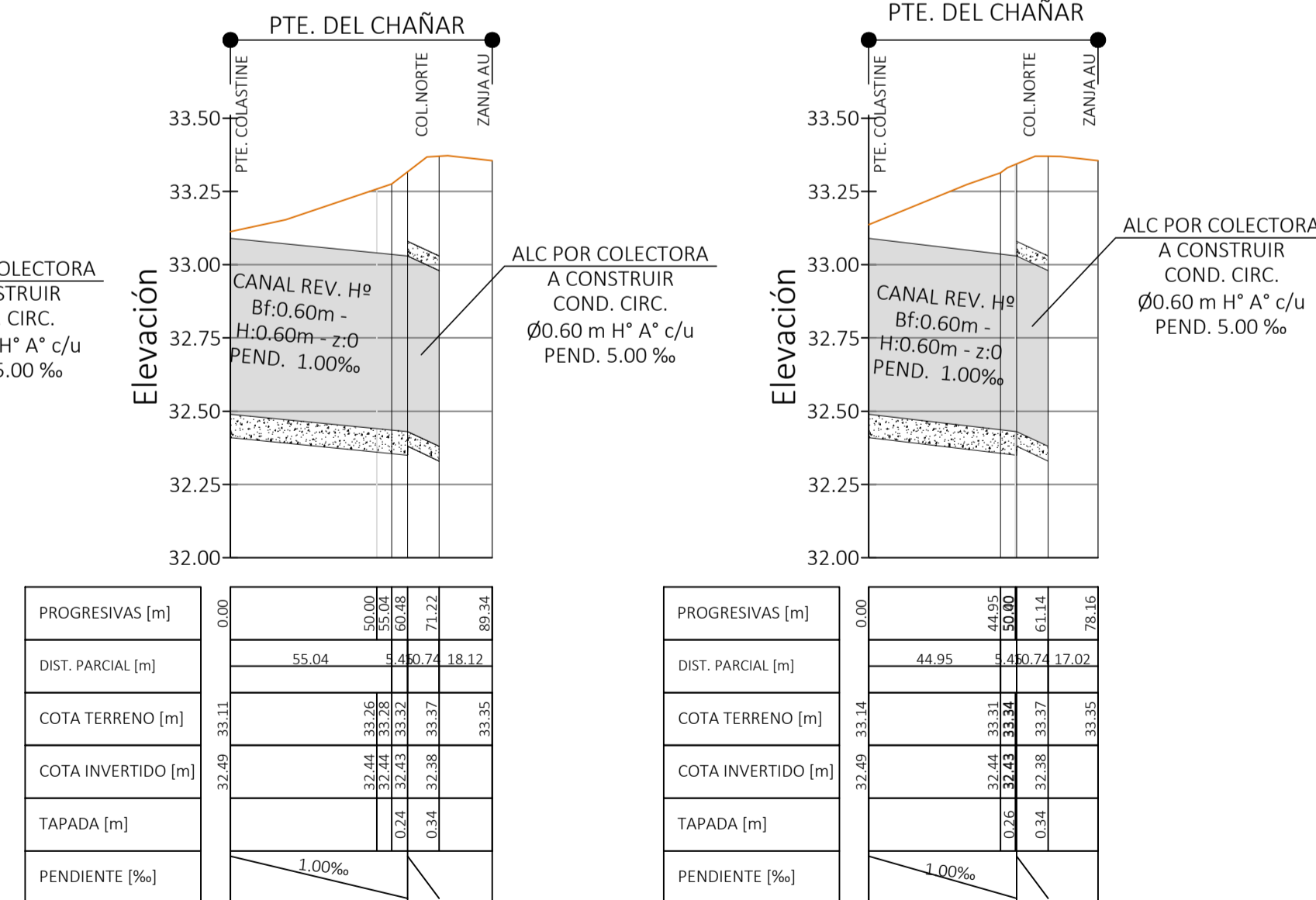
Perfil Longitudinal Ramal 11 der Perfil Longitudinal Ramal 11 izq
