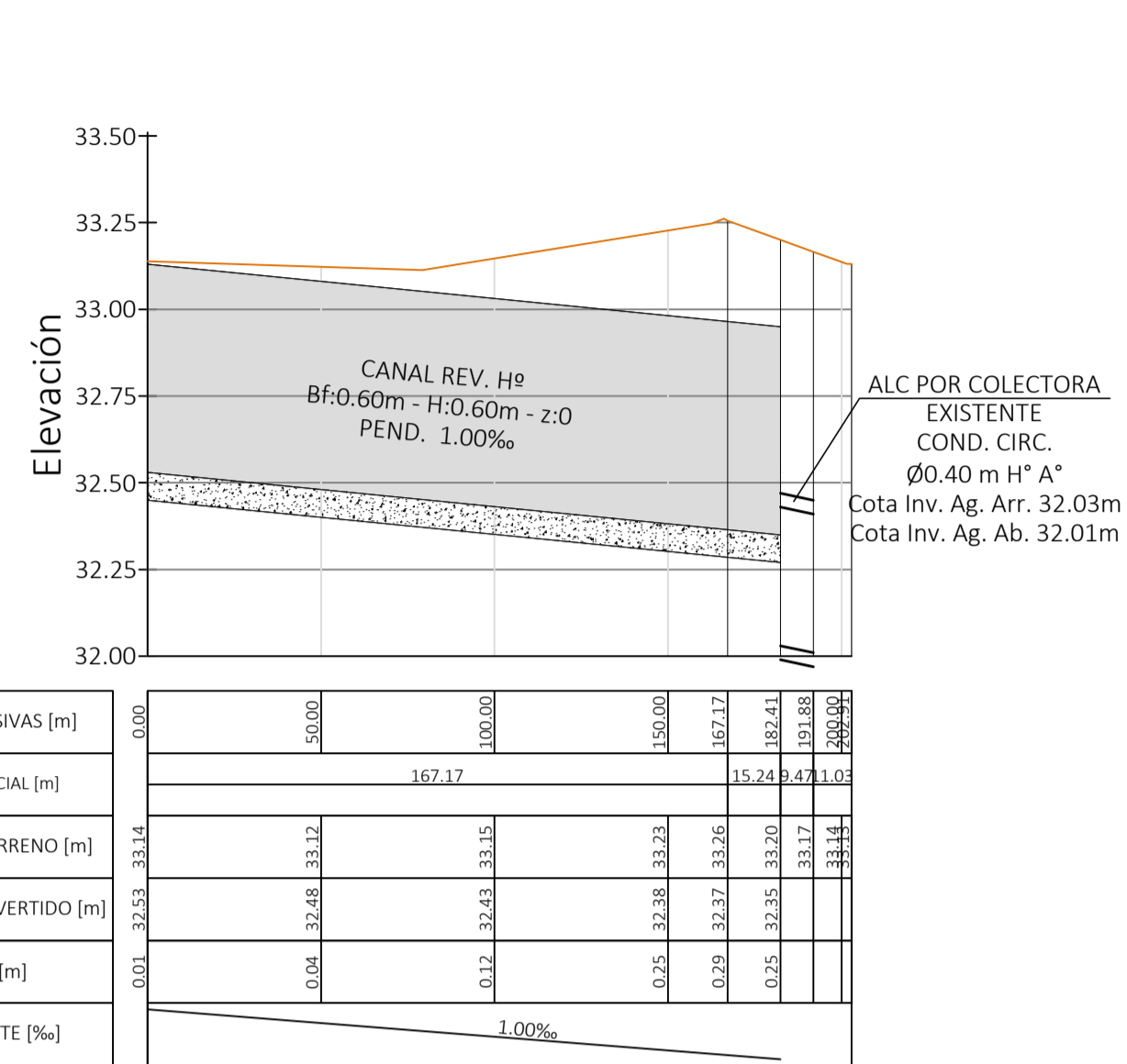
Perfil Longitudinal Ramal 12i
