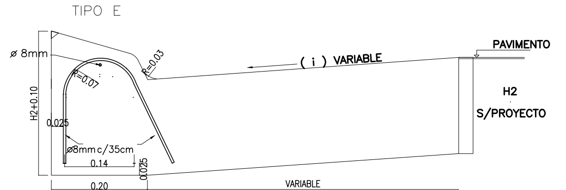
CORDON CUNETA DE ALTURA VARIABLE
